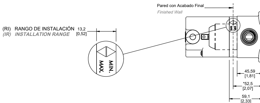
VISTA SUPERIOR (DETALLE DE INSTALACIÓN) TOP VIEW (INSTALLATION DETAIL)
